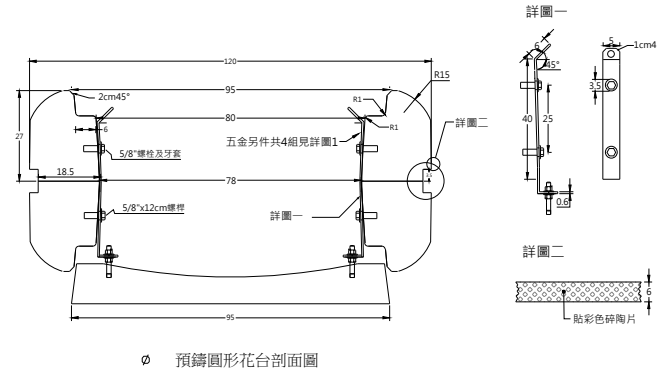
預鑄圓形花台剖面圖
