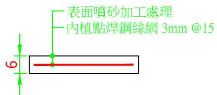
不等邊六角形預鑄混凝土板(噴砂面) TYPE-D 尺寸:邊長=25cm/TH=6cm (密鋪)
