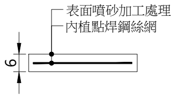
不等邊六角形預鑄混凝土板(噴砂面) TYPE-D 尺寸:邊長=25cm/TH=6cm (密鋪)
