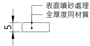
不等邊六角形預鑄混凝土板(噴砂面) TYPE-C 尺寸:邊長=15cm/TH=5cm (密鋪)
