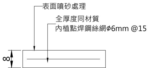
不等邊六角形預鑄混凝土板(噴砂面) TYPE-B 尺寸:邊長=50cm/TH=8cm (密鋪或疏鋪)
