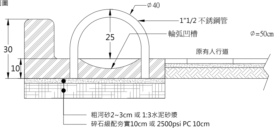
剖面圖
