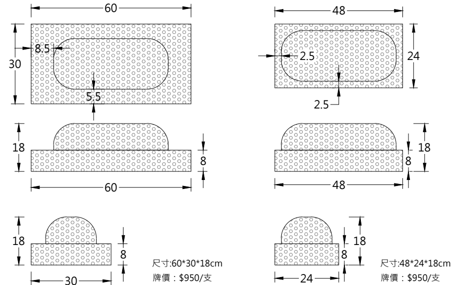
Q30 預鑄洗石子(噴砂)車輪擋
