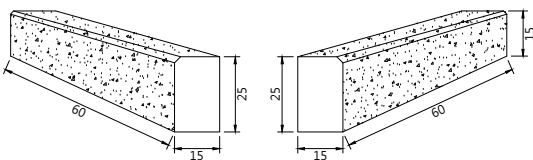
預鑄斜坡道收邊緣石(左斜)
