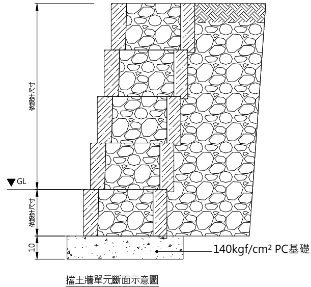
擋土牆單元斷面示意圖
