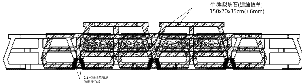
生態駁坎石單元組合示意圖
