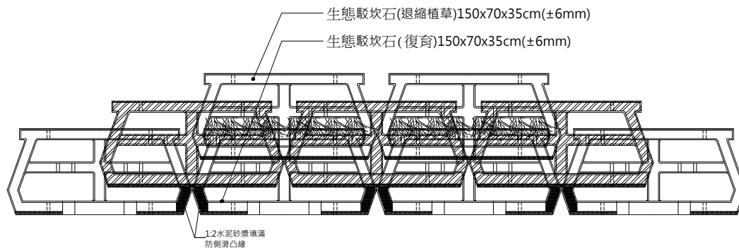
生態駁坎石(復育)單元組合示意圖
