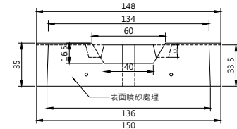
復育駁坎石 TYPE A 規格:150x70x35cm
