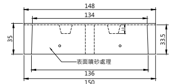
駁坎石 TYPE B 規格:150x70x35cm(±1cm) 牌價:$8700/M2
