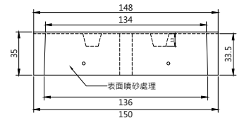
駁坎石 TYPE A 規格:150x70x35cm(±1cm)
