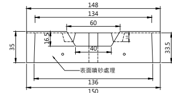
復育駁坎石 TYPE B 規格:150x70x35cm 牌價:$8700/M2
